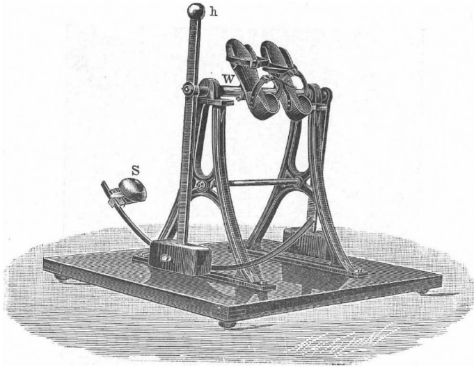
Abb. 4: Krukenberg'scher Apparat „Fußbeugen und -strecken mit Pendelantrieb“
