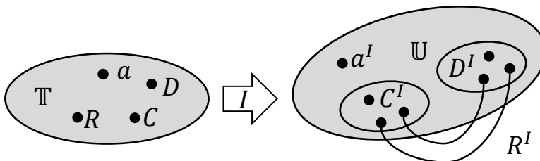
Bild 27: Interpretation einer DL-Theorie nach [123]
