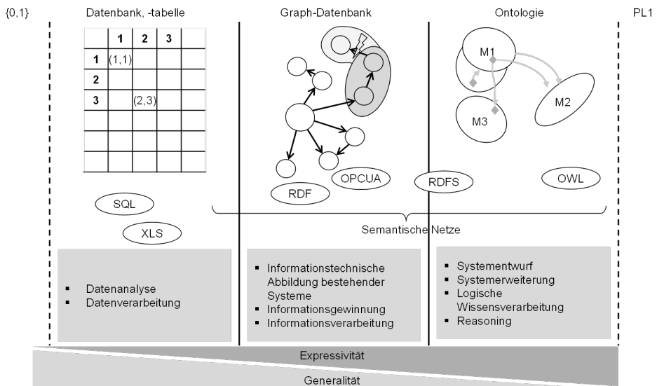
Bild 44: Semantischer Navigator zur Bestimmung der notwendigen Repräsentationsform
