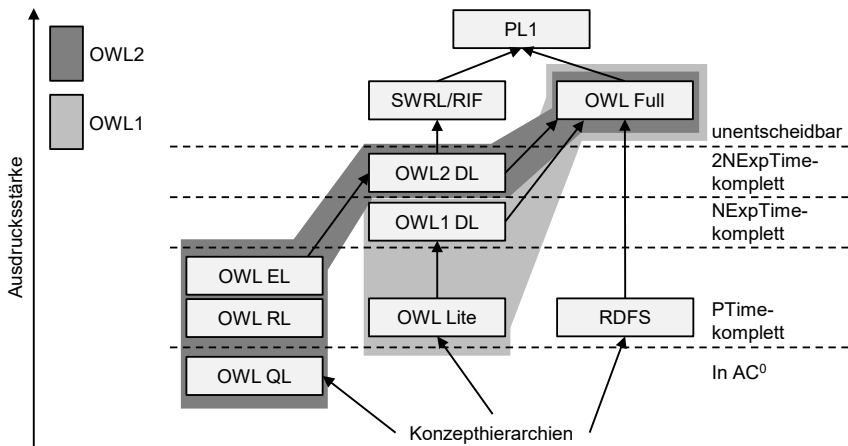
Bild 32: OWL-Sprachvarianten und Komplexitätsklassen, nach [113, 131]
