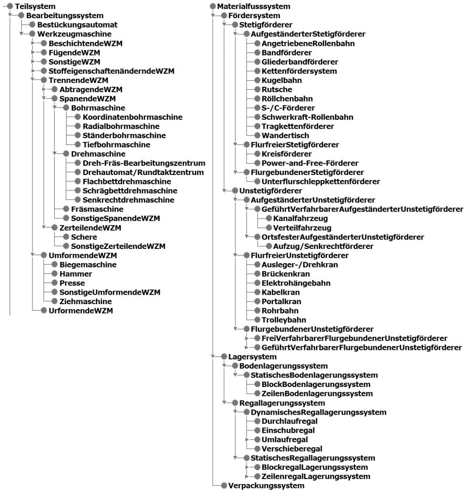
Bild 73: Klasse Teilsystem einschließlich ausgewählter Unterklassen (links) und Klasse Materialflusssystem (rechts), Screenshot aus Protégé [Si]
