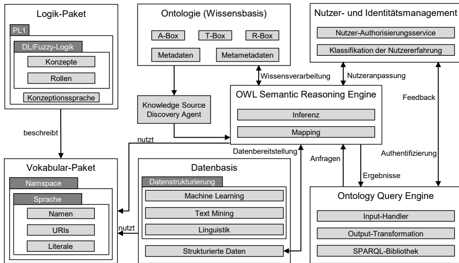
Bild 66: Aufbau des entwickelten Wissensmanagement-Frameworks, nach [S4]
