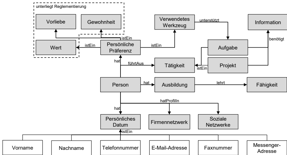
Bild 61: Meta-Modell zur Beschreibung der Mitarbeiter
