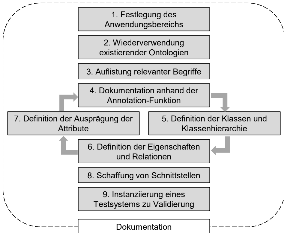
Bild 52: Vorgehensweise zur Erstellung von Meta-Ontologien [S1]
