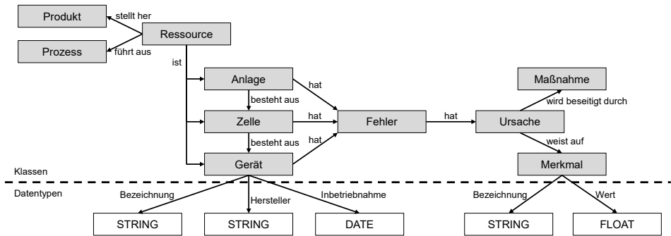
Bild 38: Ontologiebasierte Repräsentation von Fehler-Ursache-Beziehungen von Produktionsanlagen, nach [201]
