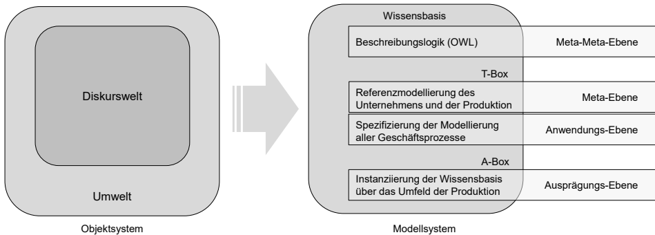
Bild 43: Darstellung des Unternehmenskontextes auf mehreren Ebenen
