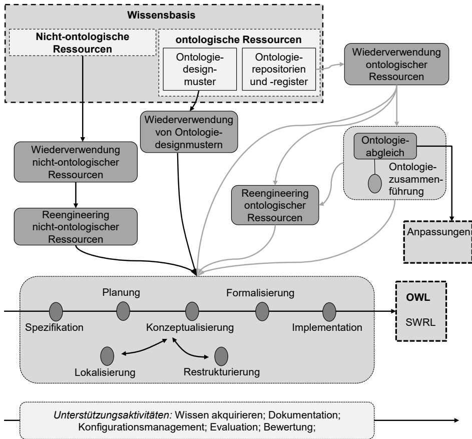
Bild 53: Ermittlung der Vorgehensweise zur Kontextanpassung, nach [278] und [S2]
