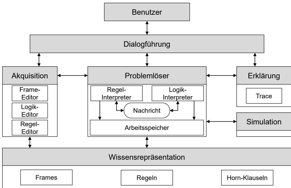
Bild 35: Struktur und Komponenten von MOPLAN, nach [192]
