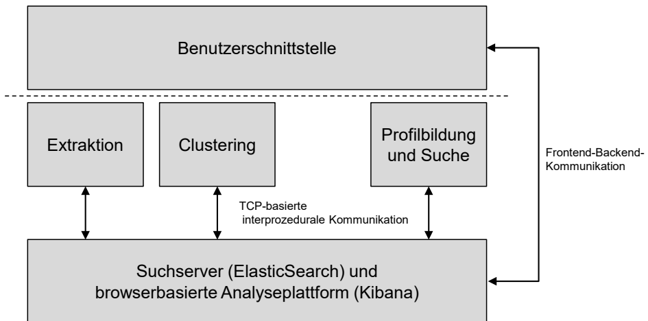
Bild 70: Architekturübersicht des Knowledge Source Discovery Agents [S8]
