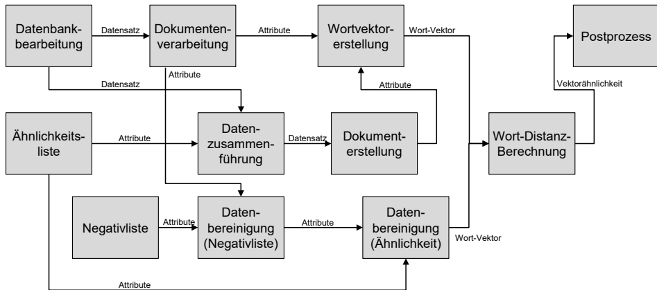
Bild 71: Empfehlungssystem zur Bereitstellung von relevanten Informationen [S9]
