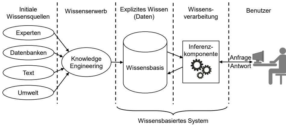
Bild 23: Struktur eines wissensbasierten Systems, in Anlehnung an [37]
