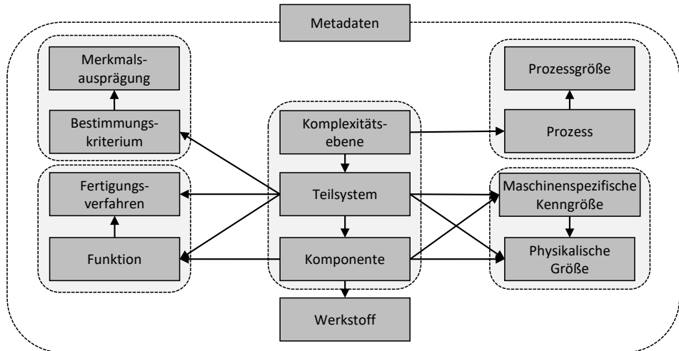
Bild 64: Metadaten-Ontologie zur Abbildung des Produktionsumfelds [Si]
