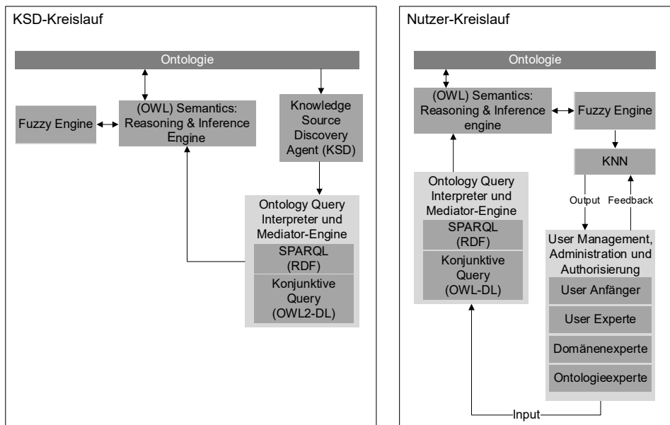
Bild 67: Ontologiekreislauf aus KSD-Sicht (links) und Nutzersicht (rechts), nach [S4]
