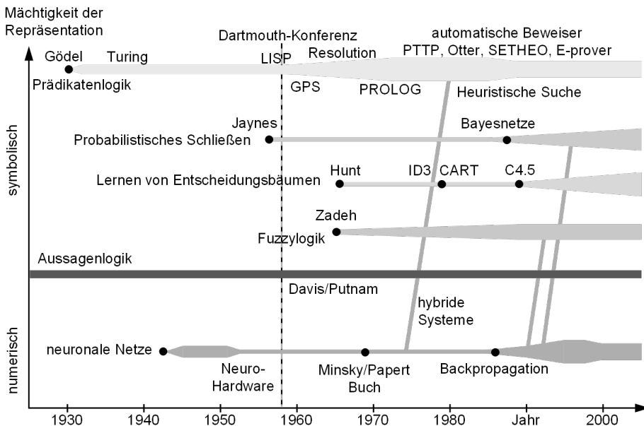
Bild 22: Entwicklung der Wissensverarbeitung in der Informatik [37]
