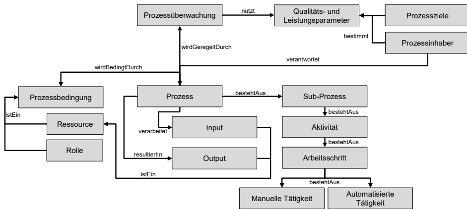
Bild 59: Generisches Prozessmodell, aufbauend auf [293]
