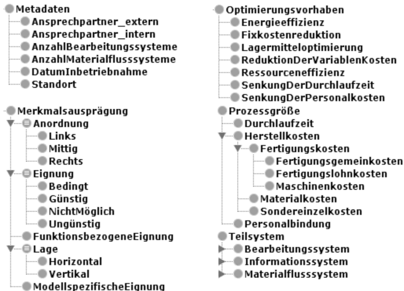
Bild 76: Partielle Darstellung von Metadaten, Merkmalsausprägung, Optimierungsvorhaben und Prozessgröße, Screenshot aus Protégé [S1]
