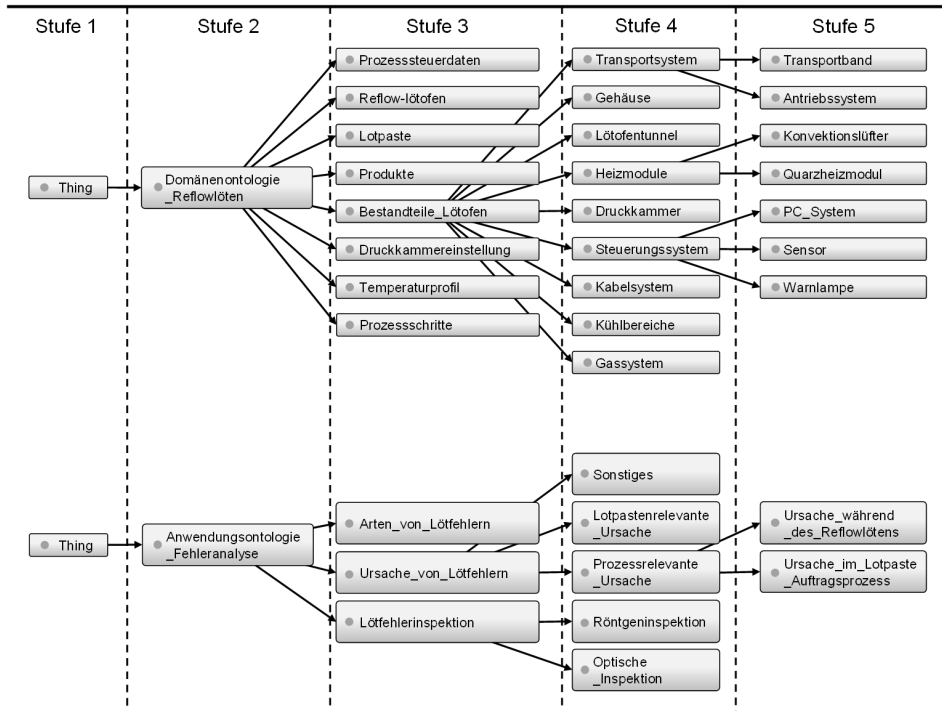
Bild 72: Ontologiehauptklassen der Modellierung des Elektronikfertigung
