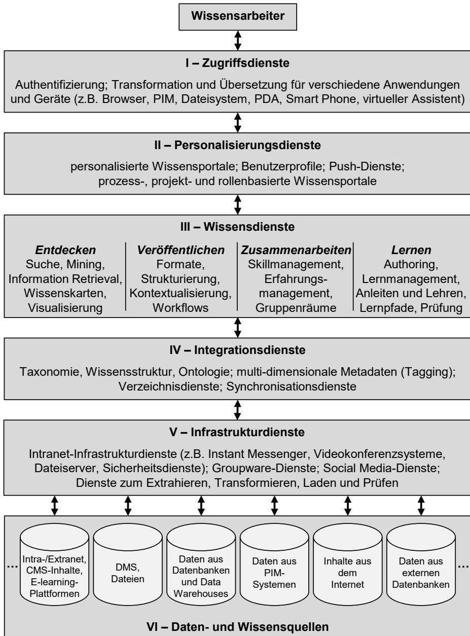
Bild 24: Architektur eines Wissensmanagementsystems, nach [51]
