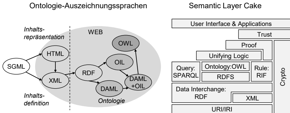
Bild 31: Entwicklung der Ontologie-Auszeichnungssprachen (links, nach [128]) und Semantic Layer Cake (rechts, nach [129])
