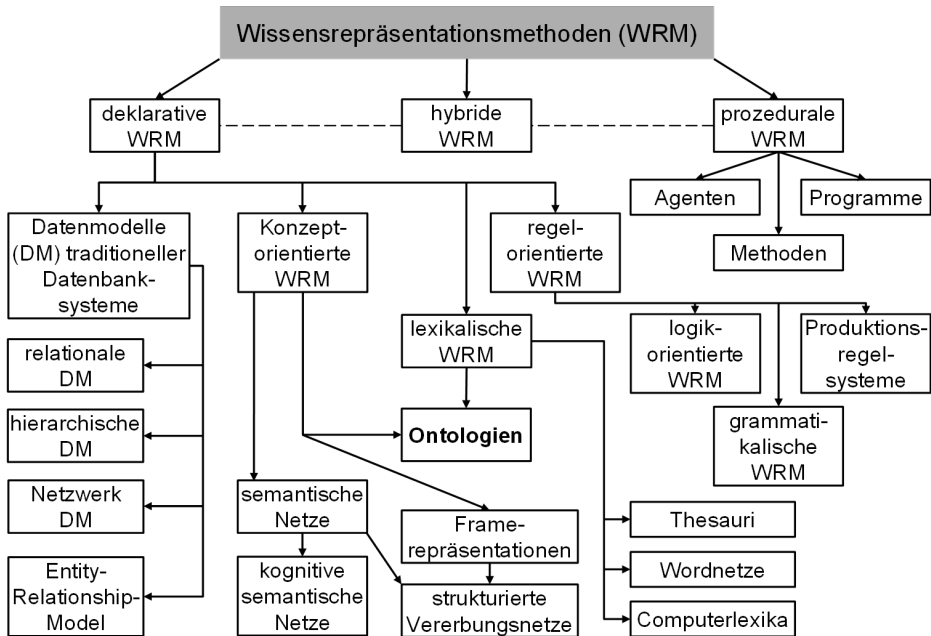
Bild 25: Überblick über Methoden der Wissensrepräsentation [104]
