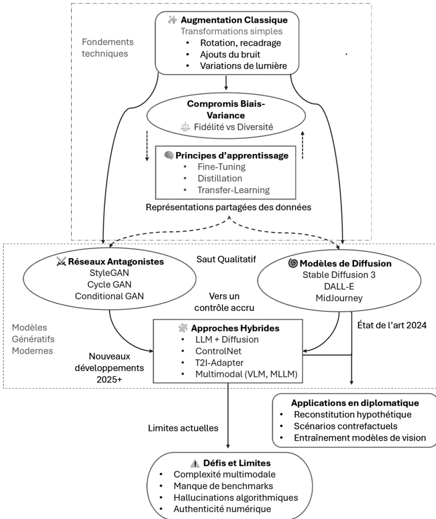
Fig. 1 : Écosystème conceptuel de la génération synthétique. La gestion du compromis biais-variance, un enjeu central pour les corpus historiques, en raison de sa quantité limitée, s'appuie sur des fondements comme l'augmentation de données et le transfert de connaissances. Ces bases techniques soutiennent la trajectoire évolutive des modèles génératifs (GANs, Diffusion, 2020–2024) vers les approches hybrides mêlant modèles de langage et de vision (2025+). L'ensemble de cette évolution présente à la fois des applications pour les sciences historiques et des défis pour la critique documentaire.
